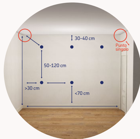
Schema dei fori per intercapedini sp. \geq 6 cm
