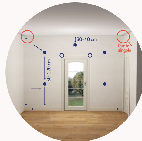
Schema dei fori per intercapedini sp. \geq 6 cm. Dettaglio porta
