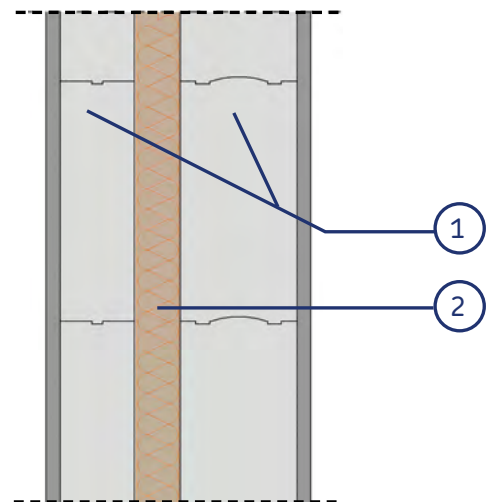
1. Pareti in blocchi di calcestruzzo cellulare autoclavato 2. URSA TERRA 66
