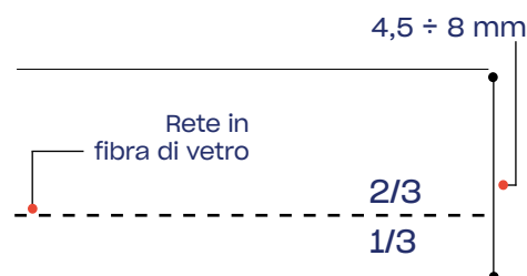
Disegno 3
